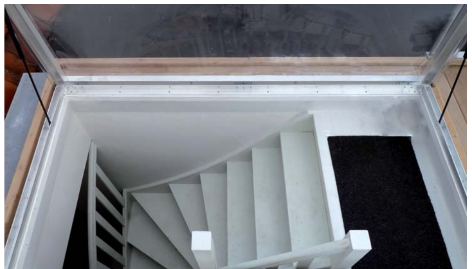
Accès toiture, cadre aluminium avec vérins à gaz, 3 poignées
