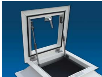
Dachausstieg, Aufsatzkranz PVC, Lüfterrahmen PVC mit Klinke und Teleskoprohre
