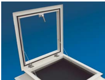
Notluke, Aufsatzkranz PVC, Lüfterrahmen PVC mit Klinke und Ketten
